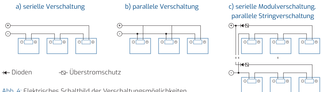
Abb. 4: Elektrisches Schaltbild der Verschaltungsmöglichkeiten
